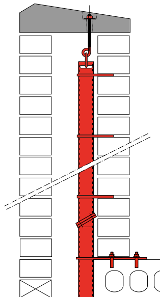
Type 2 Met voetplaat speciaal voor kanaalplaatvloeren
