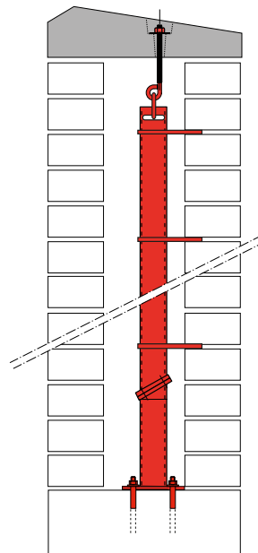
Type 3 Met voetplaat
