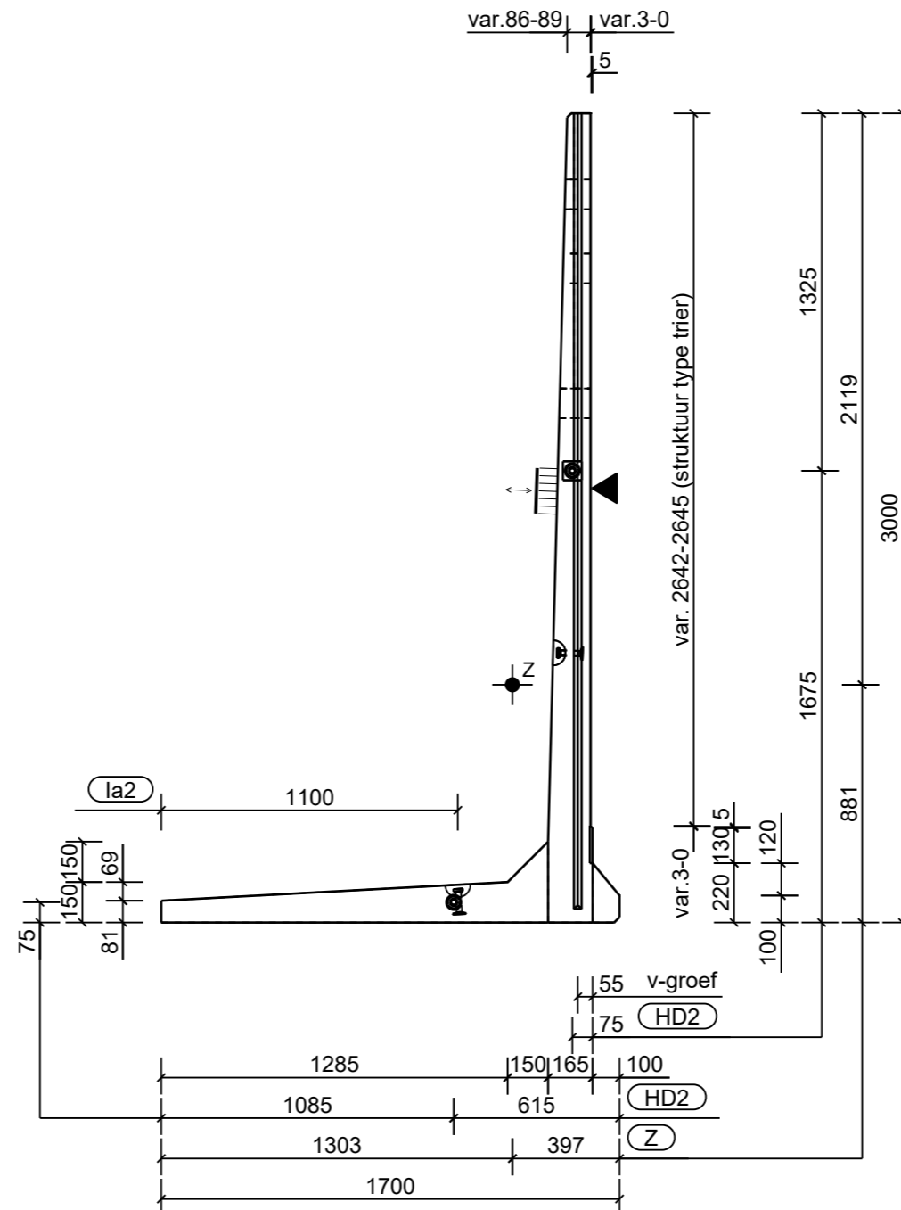
Zijaanzicht B
