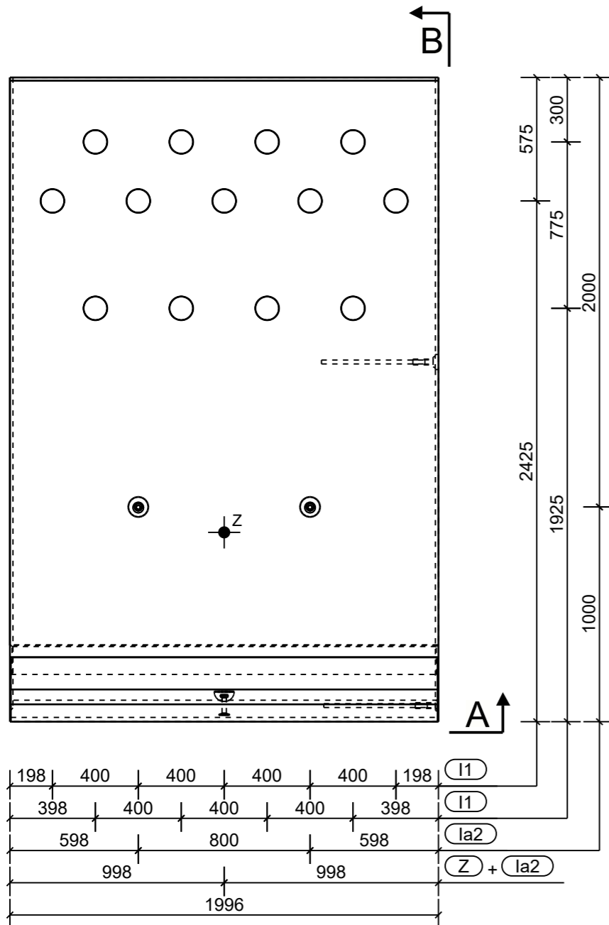
Aanzicht stortzijde
