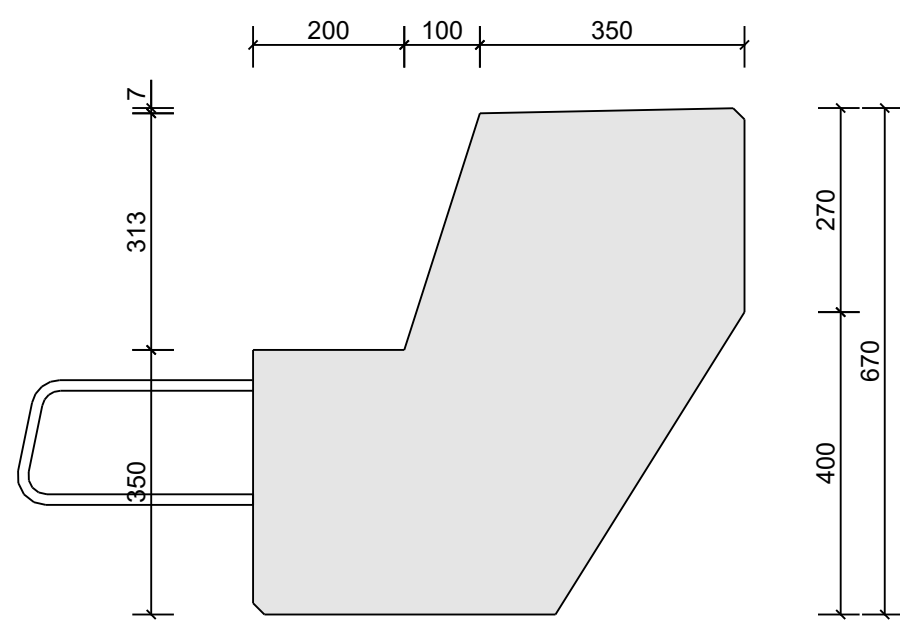
H=350/670
