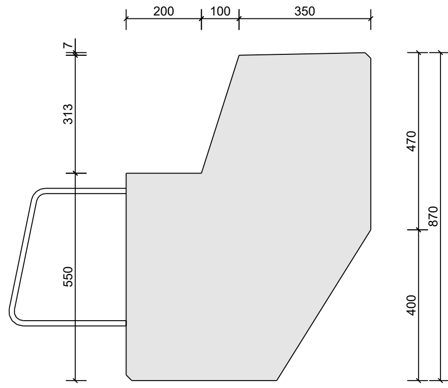
H=550/870
