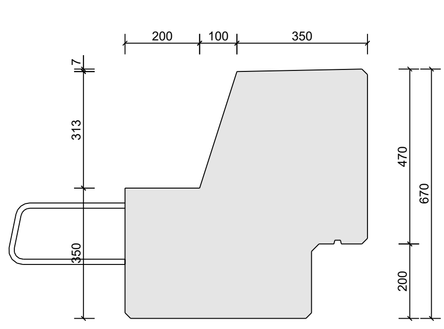
H=350/670
