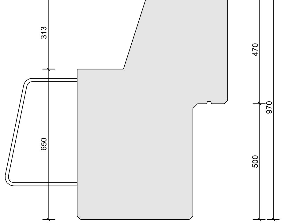
H=650/970
